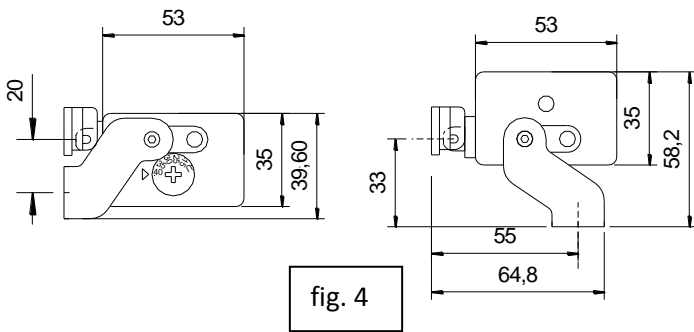
Installazione serramento a sporgere - top hinged installation
